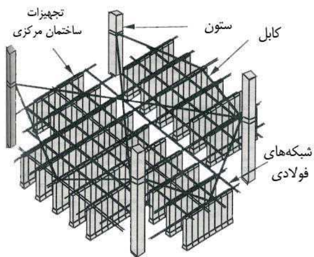
شکل ۵-۴- سامانه مهاربندی کابل افقی
