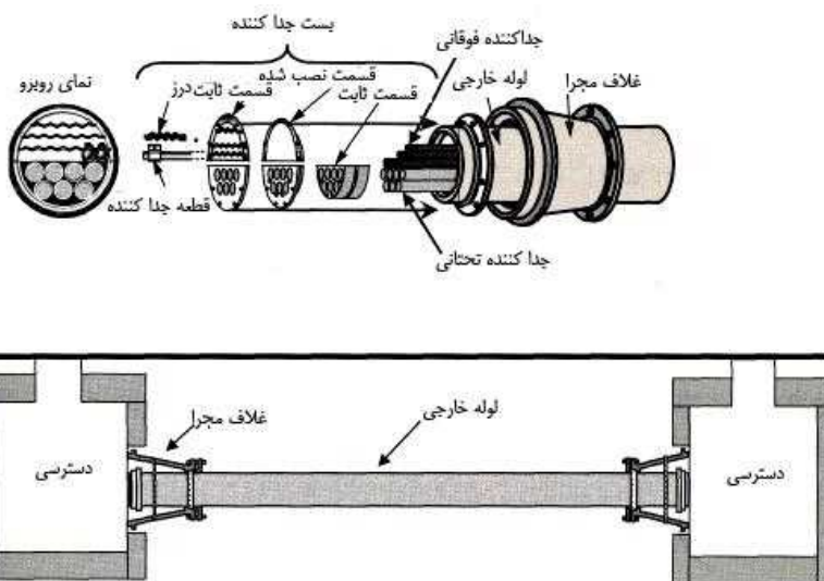
شکل ۵-۲۰ روش اجرای جدید مجرای انتقال کابل
