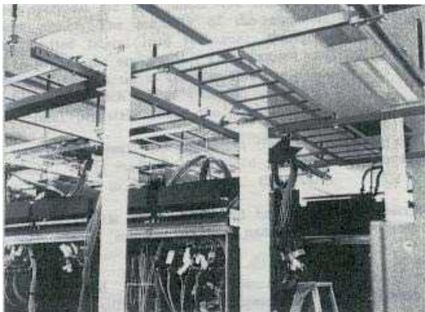
شکل ۵-۳- پایدارسازی جانبی ردیف‌های تجهیزات
