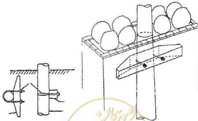
شکل ۱۵-۵- جزئیات بهسازی پایه‌های خطوط هوایی مخابراتی
