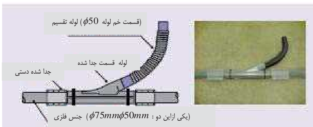
شکل ۵-۱۸- انشعاب انعطاف پذیر از مجرای اصلی
