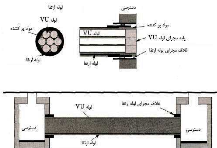
شکل ۵-۱۹ روش اجرای قدیمی مجرای انتقال کابل
