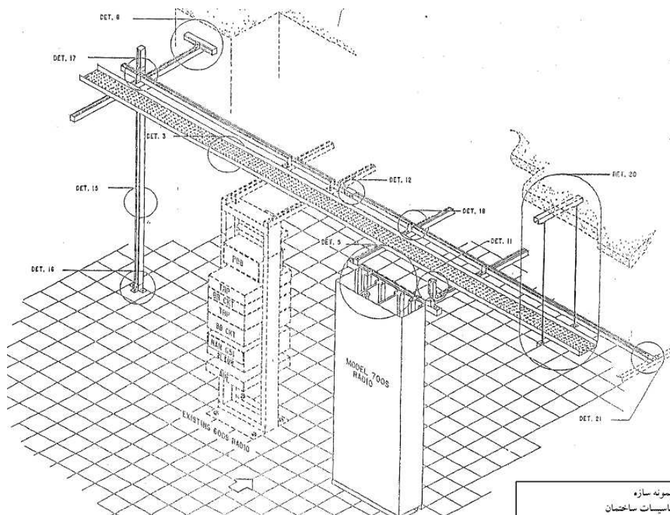
شکل ۵-۲- پایدار سازی تجهیزات رادیو به کف و دیوارها
