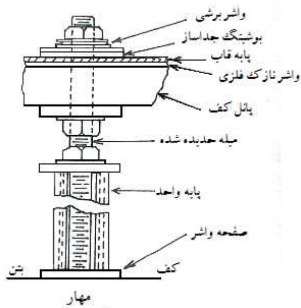
شکل ۵-۶- پیچ مهاري که از کف کاذب عبور می کند
