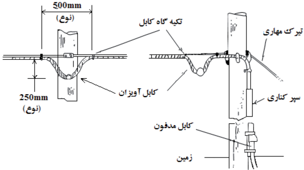
شکل ۱۴-۵- انعطاف پذیری اتصال کابل هوایی
