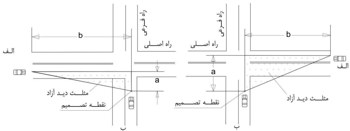
مثلث دید آزاد برای رویت تَرَافِیکی که از سمت چپ می‌رسد
