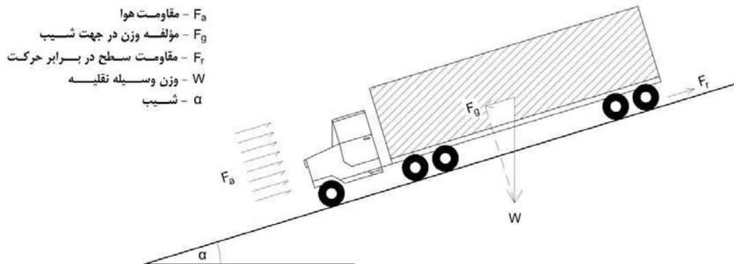
شکل ۵-۱۹- نمایش کامیون و نیروهای وارده در سرازیری
