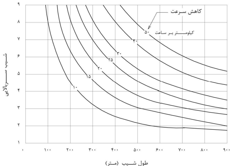
شکل ۵-۹- رابطه بین مقدار و طول بحرانی شیب برای مقادیر مختلف کاهش سرعت برای کامیون (سرعت اولیه ۱۱۰ کیلومتر در ساعت)
