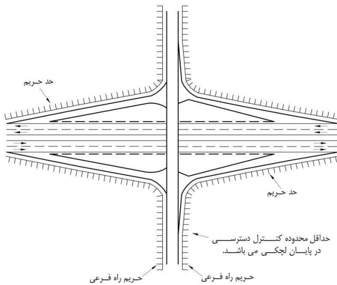
ت- محدوده کنترل دسترسی در تبادل لوزی
