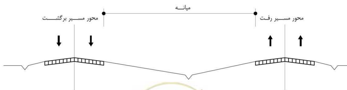
شکل ۴-۶- مرحله اول ساخت یک راه چند خطه جداشده
