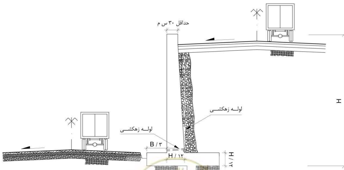
شکل ۶-۱۳ - دیوار حایل وزنی
