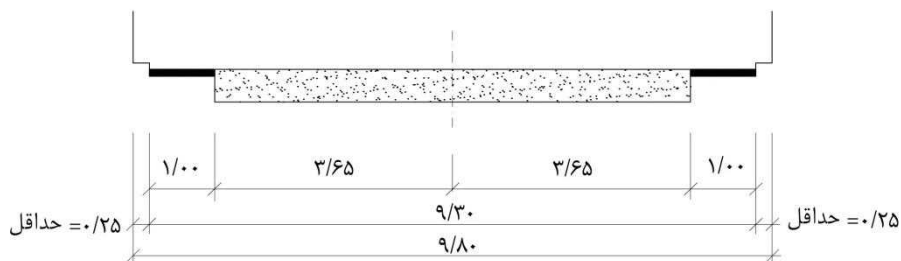
تونل دو طرفه با شانه یک متری بدون پیاده رو اضطراری
