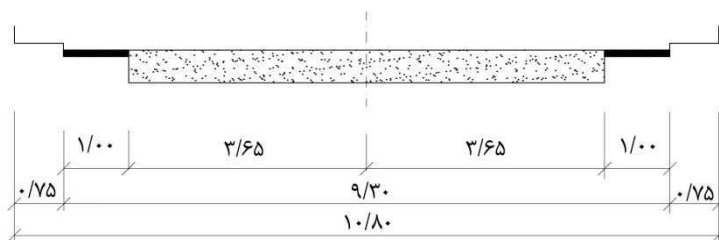
تونل دو طرفه با پیاده رو اضطراری و شانه یک متری
