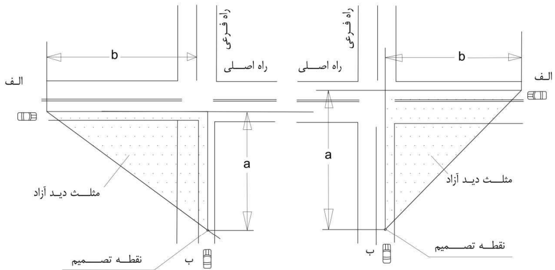
مثلث دید آزاد برای رویت تَرَافِیکی که از سمت چپ می‌رسد
