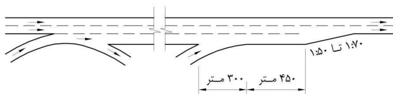
ه- حذف خط کمکی بعد از تبادل
