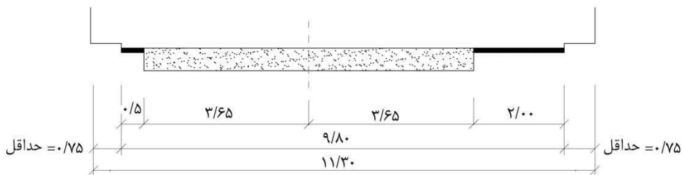
تونل یکطرفه با نوار توقف اضطراری
