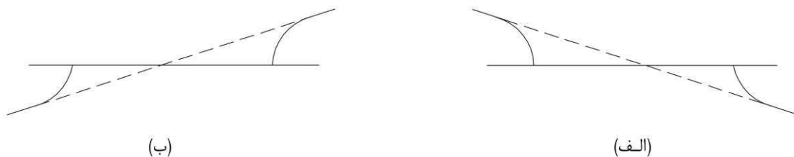
شکل ۸-۱۷- نحوه اصلاح مسیر در تقاطع‌های با زاویه تند
