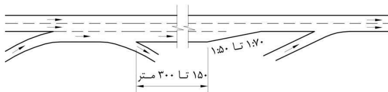
د- حذف خط کمکی در طول تبادل
