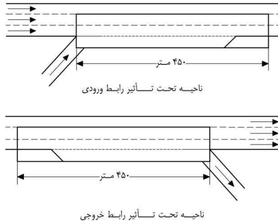
شکل ۷-۸- ناحیه تحت تأثیر رابط‌های ورودی و خروجی در محل تلاقی با آزادراه‌ها
