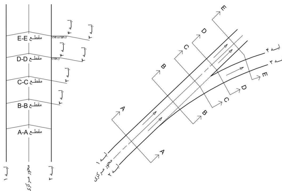
شکل ۸-۲۹- نحوه تأمین برابندی در پایانه- جداسازی از خط مستقیم
