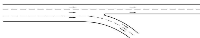
شکل ۹-۲۹- حالت‌های متداول خروجی‌های چند شاخه‌ای
