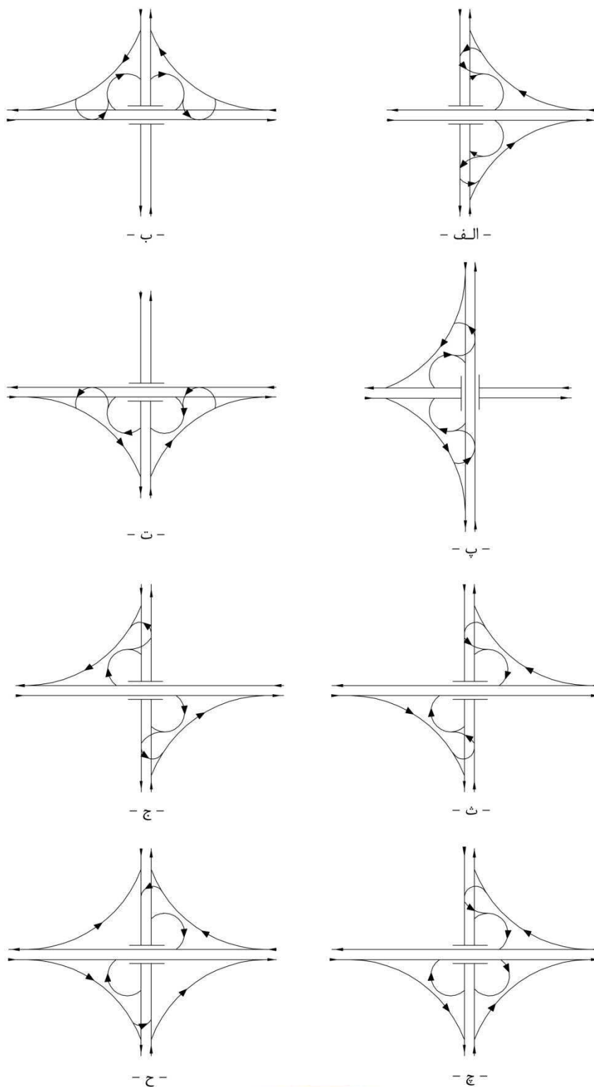
شکل ۹-۹- نمونه طرح‌های ورودی و خروجی تبادلهای نیمه‌شبدری
