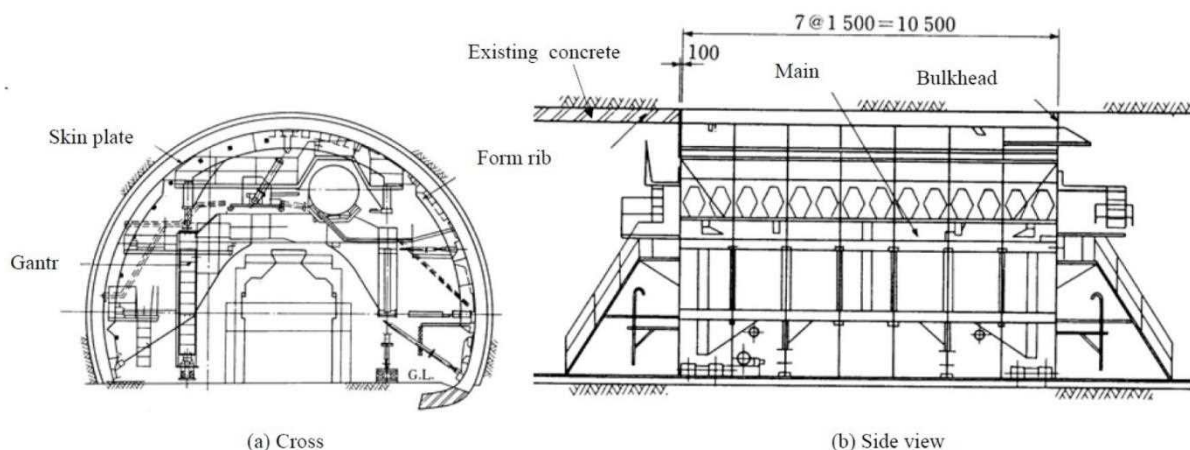
شکل ۶-۱۴- نمونه ای از قالب متحرک
