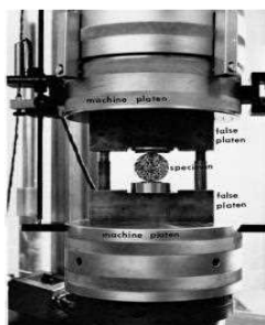
شکل ۳-۴- آزمایش برزیلی جهت تعیین مقاومت کششی
