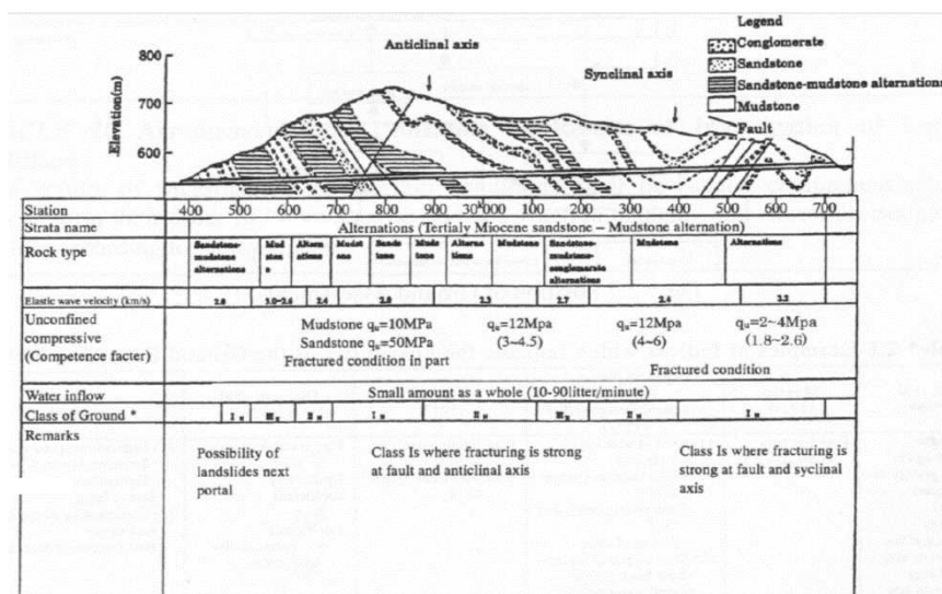
شکل ۲-۲ - نمونه‌ای از مشخصات زمین‌شناسی طولی
