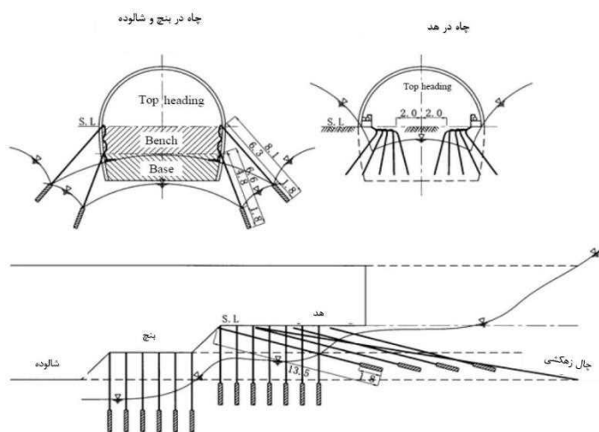
شکل ۶-۳۲- نمونه از چاه نفوذی (well point) غرق شده در تونل
