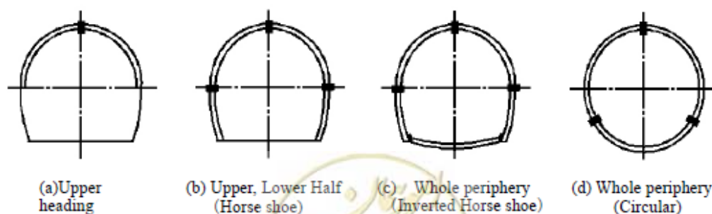
شکل ۵-۹- a (هدینگ)، b (نیمه بالا و پایین (نعل اسبی))، c (پیرامونی (نعل اسبی کفبنددار)) و d (پیرامونی (داپروی))
