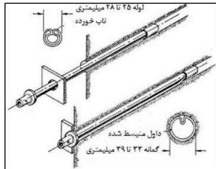
شکل ۵-۸ - نمونه‌ای از راکبالت اصطکاکی
