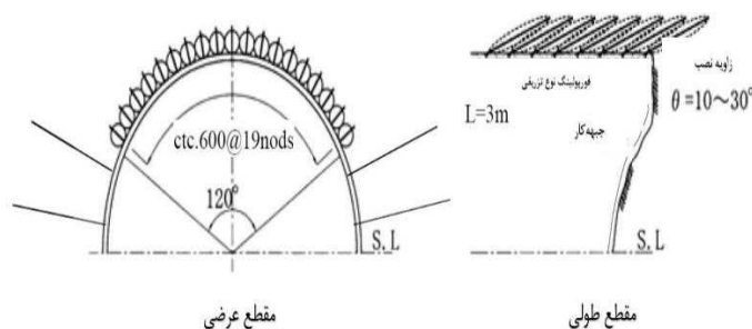
شکل ۶-۲۴- نمونه از فورپولینگ نوع تزریقی
