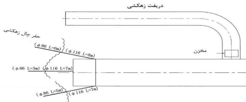
شکل ۶-۳۱- نمونه‌ای استفاده ترکیبی از دریفت زهکشی و حفاری زهکشی
