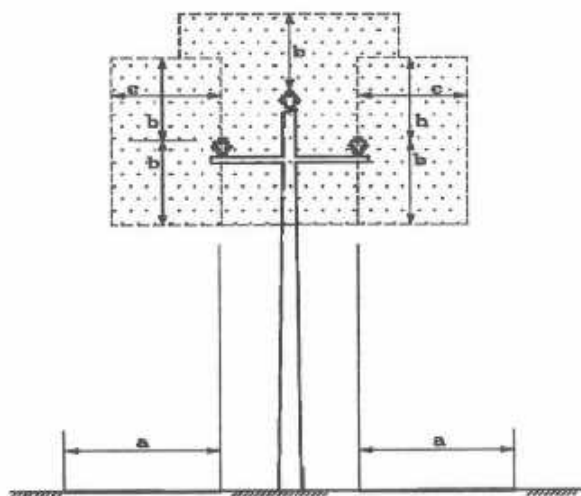
شکل ۲-۱۹- خط هوایی فشار متوسط (۱۱، ۲۰ و ۳۳ کیلو ولت)
