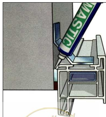
شکل ۱۲-۵۵- استفاده از نبشی از نبشی دو خم‌دار برای سهولت انجام درزبندی
