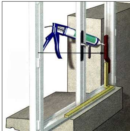
شکل ۱۲-۵۸- همپوشانی بتانه با اسفنج در دربندی
