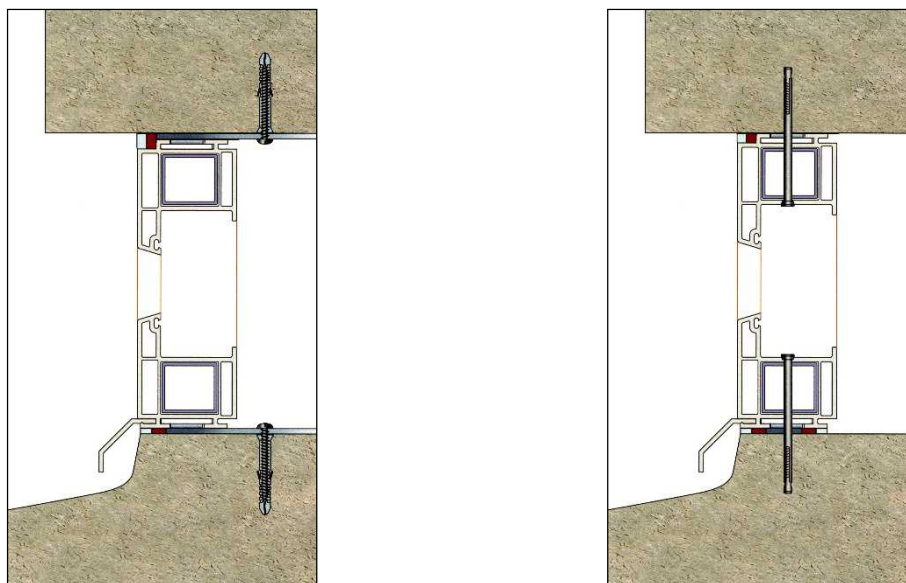
شکل ۱۲-۴۳- نصب غیر مستقیم پنجره و در به دیوار توپر بنایی یا بتنی توسط بست و رول پلاگ
