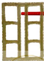
شکل ۱۲-۴۷- لزوم درگیر شدن رول‌پلاگ با حداقل دو بدنه بلوک سفالی
