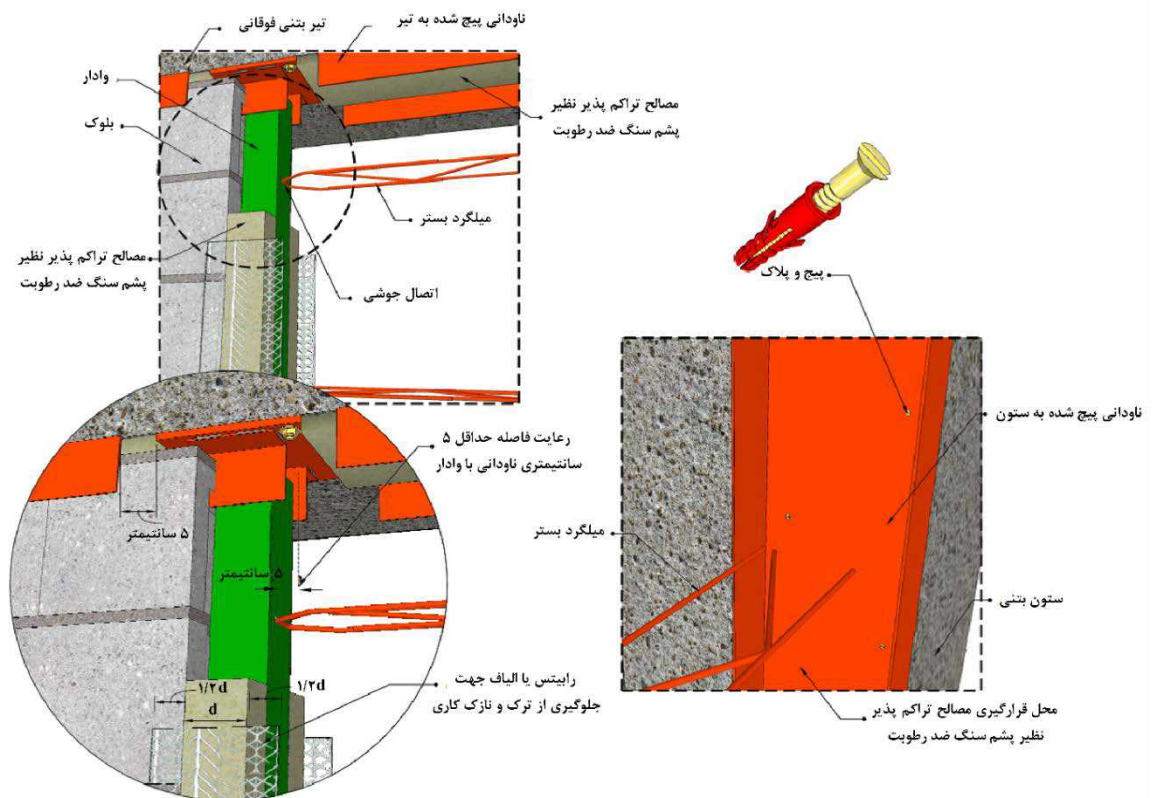
شکل ۱۱-۷- اجرای عایق پشم سنگ و مش الیاف یا رابیتس بر روی وادیار
