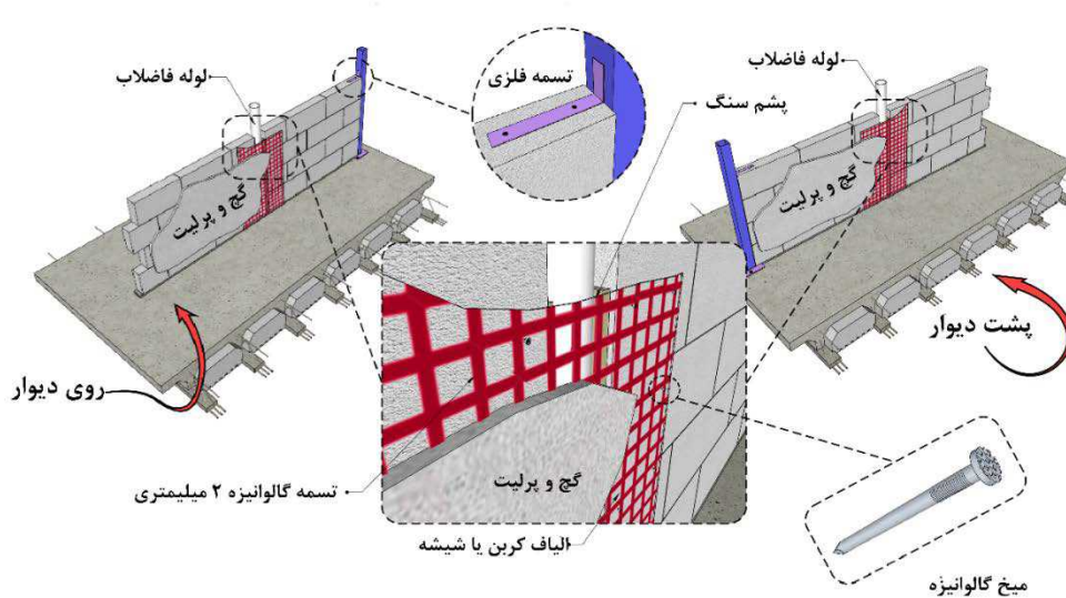
شکل ۱۱-۱۰- اجرای مش الیاف بر روی شکاف سرتاسری ایجاد شده در دیوار به وسیله لوله های تاسیساتی جهت تامین پایداری دیوار و جلوگیری از ترک خوردن اندود گچی
