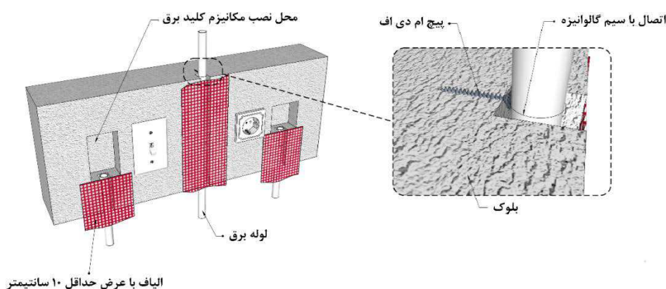
شکل ۱۱-۹- اجرای رابیتس یا مش الیاف بر روی شکاف های ایجاد شده در دیوار پیش از اجرای پوشش گچی جهت جلوگیری از ترک خوردگی اندود
