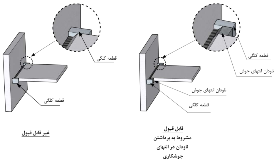
شکل ۷-۴ - شرایط پذیرش قطعه کنگی
