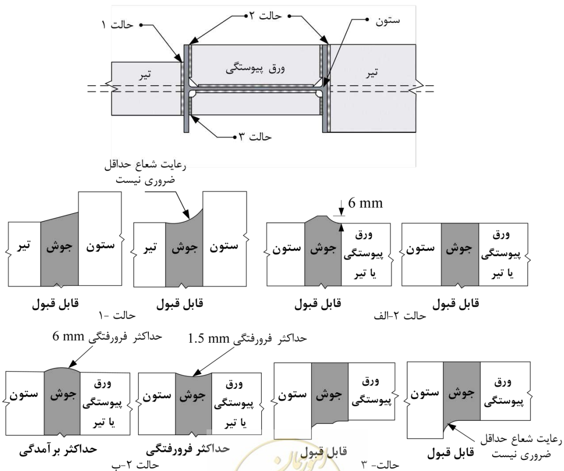
شکل ۷-۵ - وضعیت‌های قابل قبول برداشتن ورق‌های گوشواره‌ای در انتهای گوش‌های شیاری با نفوذ کامل
